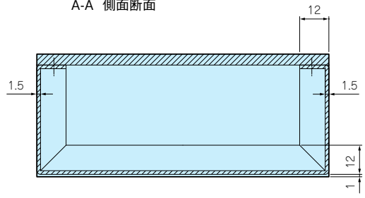
A-A 側面断面
