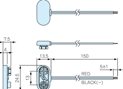
MP-TLN外観寸法図
