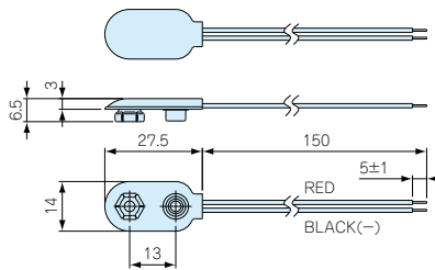
MP-1SN外観寸法図
