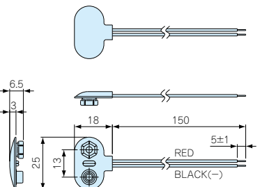
MP-TSN外観寸法図
