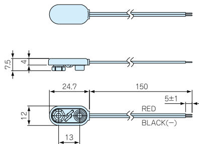
MP-1LN外観寸法図
