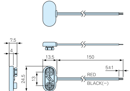
MP-TLN外観寸法図
