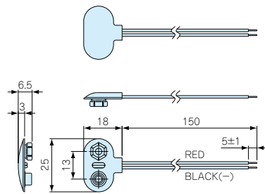
MP-TSN外観寸法図
