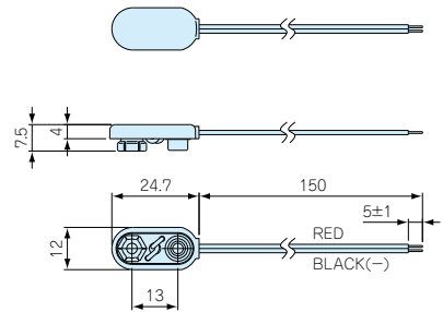
MP-1LN外観寸法図
